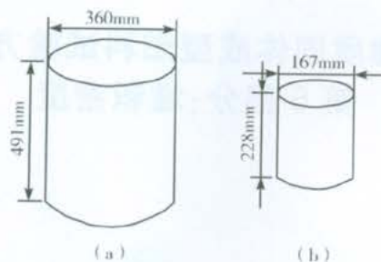
图1 测量容器示意图
